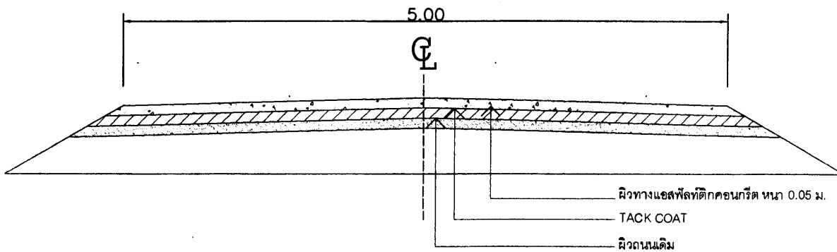
รูปตัดโครงสร้างถนน ก-ก
