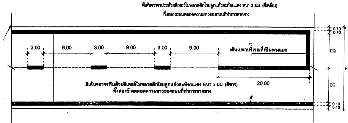
แบบขยายการตีเส้นจราจร
