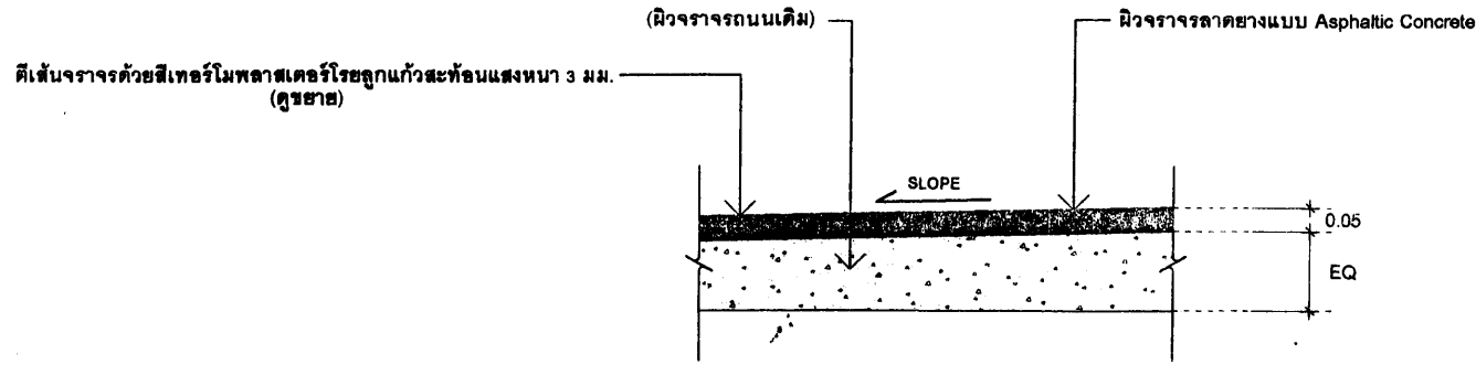
แบบขยาย ASPHALTIC CONCRETE
